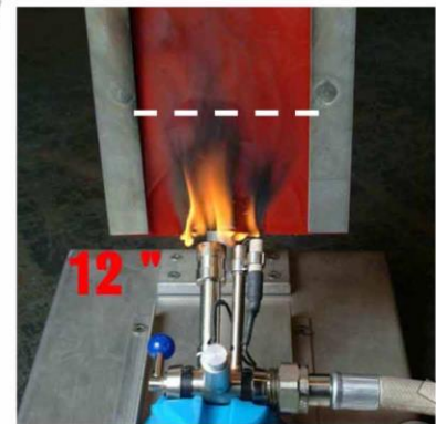
12 s – a lángmagasság határértéke (150 mm)
